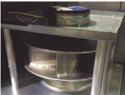
Plenum Fan with Integral ECM Motor
